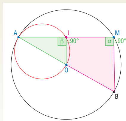
Construction avec la trace de I
